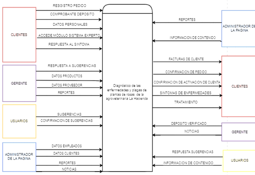
Figura 2. Diagrama de contexto
